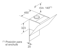
(1) Posición para el enchufe. Tener en cuenta el grosor máximo de la pared trasera. Dimensiones en mm
