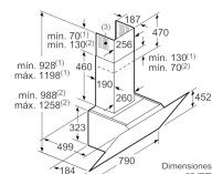
(1) Salida de aire al exterior (2) Circulación de aire (3) Salida de aire al exterior. Montar con las ranuras de la salida de aire hacia abajo. Dimensiones en mm
